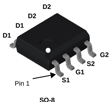
SO-8
